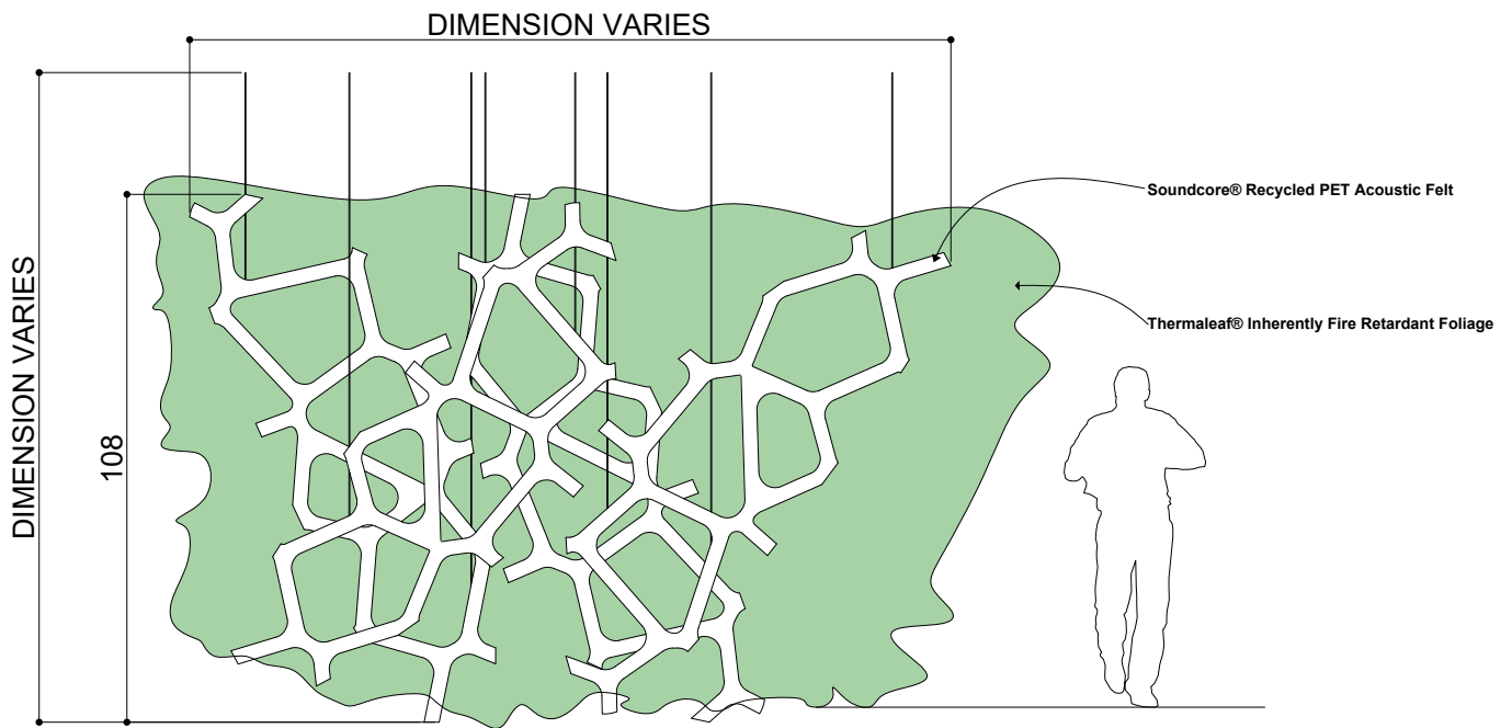
② ELEVATION 2
